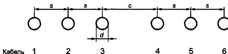
Рисунок 1 - Расположение кабелей
